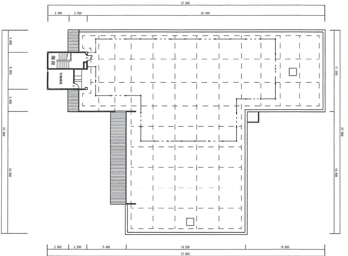
PH階平面図 S=1/200
