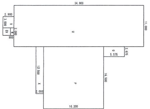
3階求積図 S=1/400
