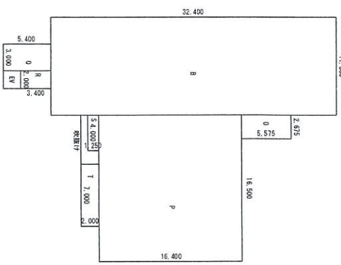
2階求積図 S=1/400
